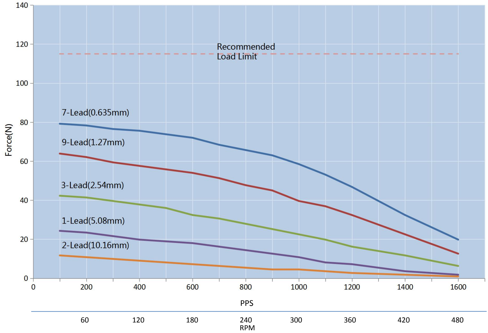
Nema 11 linear steppers(24V)
