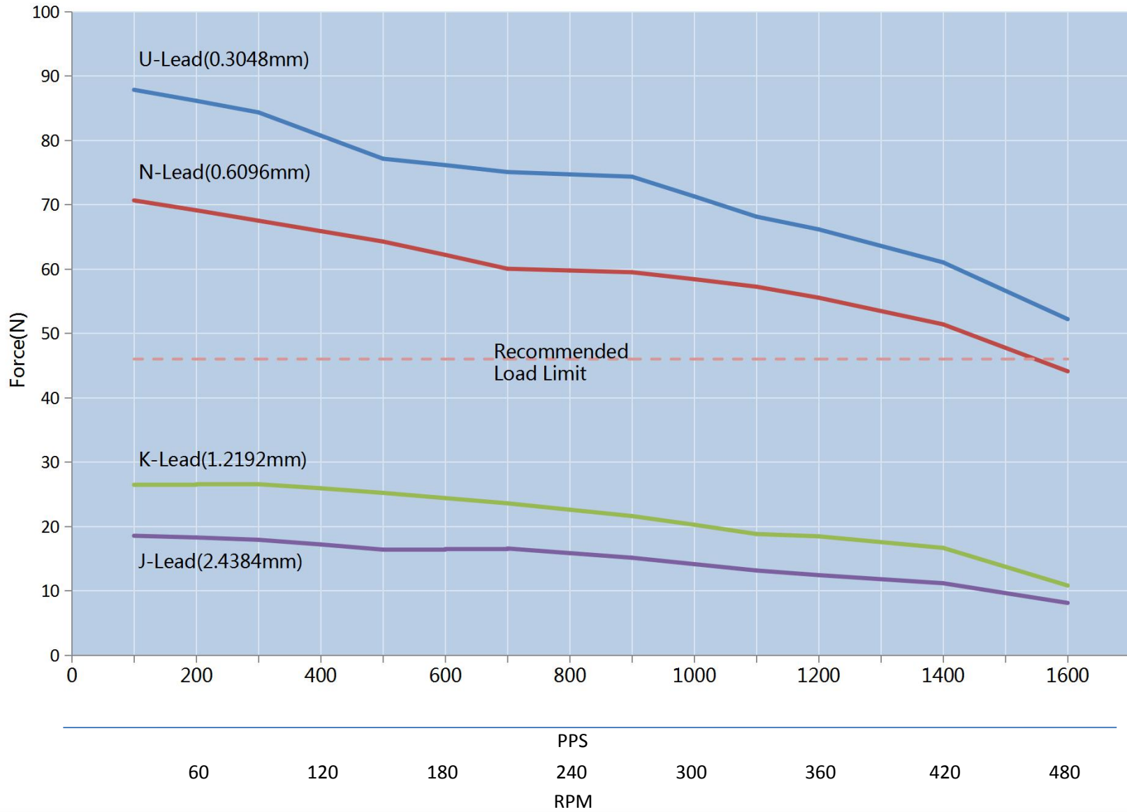
Nema 8 linear steppers(24V)
